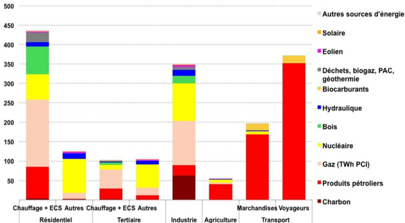
Consommation finale d'énergie en 2014 (en TWh) Source: SOeS, RTE, CEREN, SNCU
